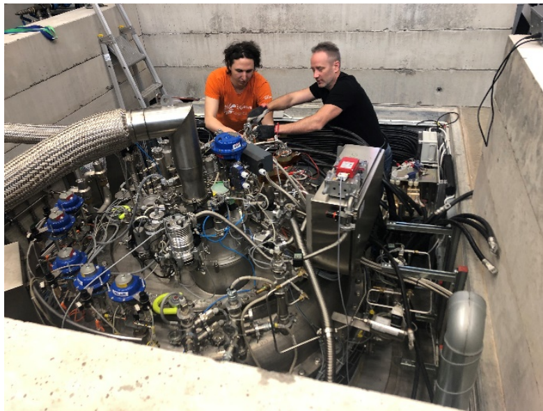
A "Gersemi" kriosztát az Uppsalai Egyetem FREIA laboratóriumában. Barna Dániel és Brunner Kristóf a nagy-áramú tápkábeleket csatlakoztatják.
